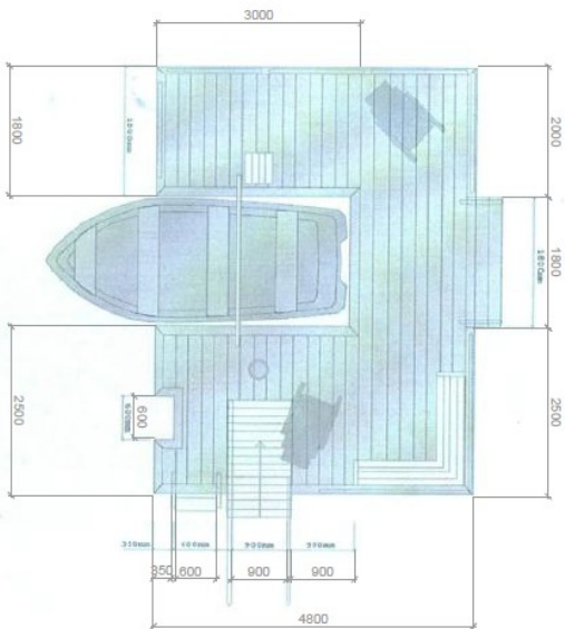
Laivu piestātnē cilvēkiem ar kustību traucējumiem. Plāns
